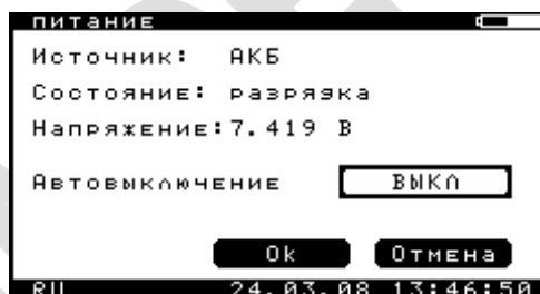
Рисунок 2.6.3.1 - Подменю «Питание»
