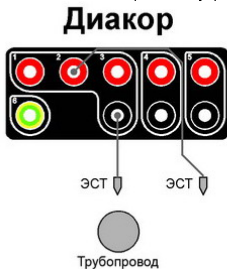
Рисунок 2.13.3.1 - Схема подключения прибора для измерений методом «ИПИ»
