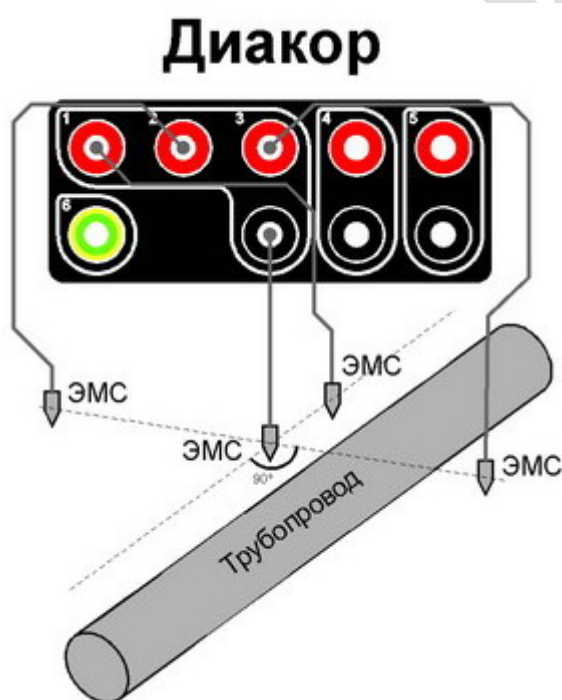
Рисунок 2.13.2.2 - Схема подключения прибора для измерений 3-х электродным методом
