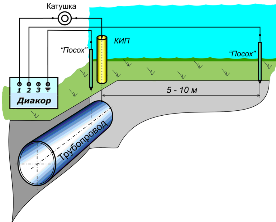
Рисунок 3.1.2.3.1.1 – Двухэлектродный метод
