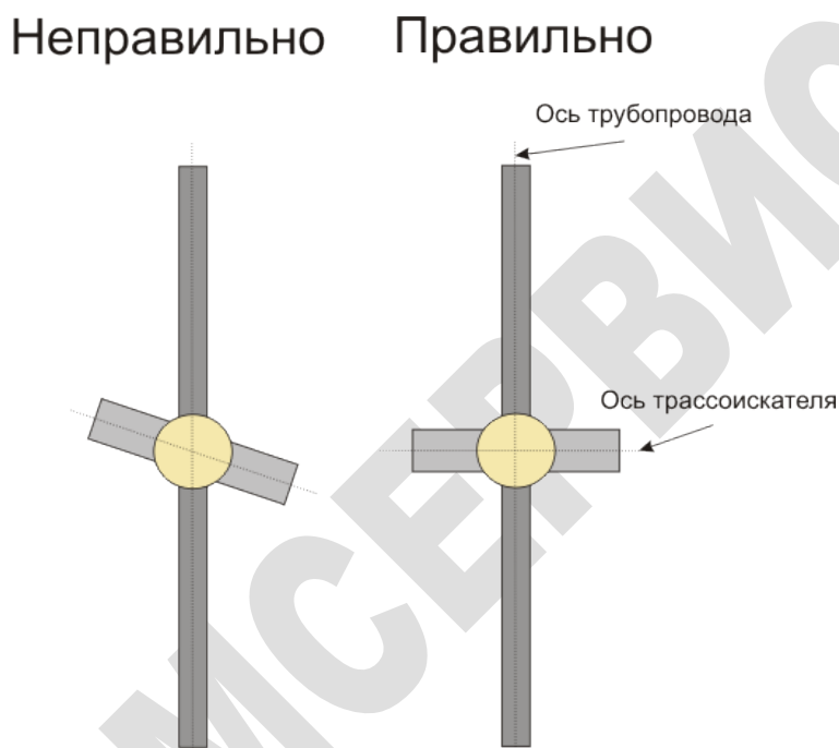
Рисунок 2.12.2.2 – Ориентация оси горизонтальных датчиков относительно оси трубопровода (вид сверху)
