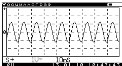
Рисунок 2.8.4.2 – Окно «Осциллограф»
