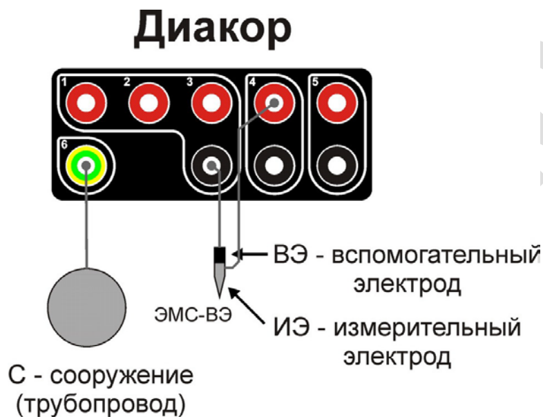
Рисунок 2.13.4.1 - Схема подключения прибора для измерений поляризационного потенциала
