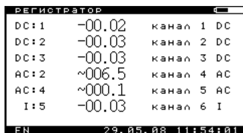
Рисунок 2.8.5.15 – Окно «Регистратор»
