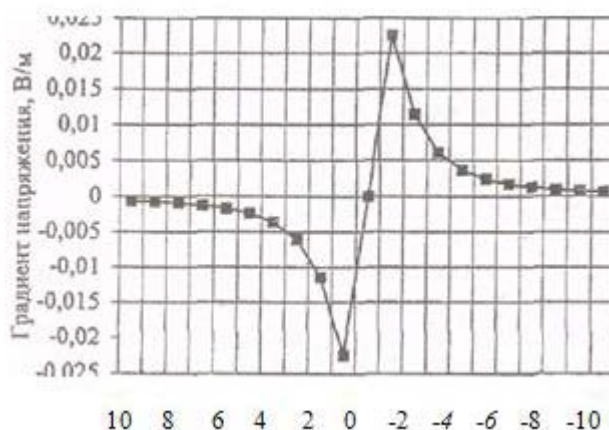
Рисунок 3.1.2.3.1.1 – Продольный градиент
