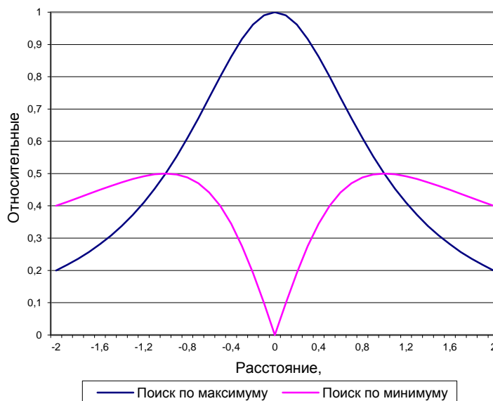
Рисунок 2.12.2.1 – Зависимость сигнала от положения оси трубопровода
