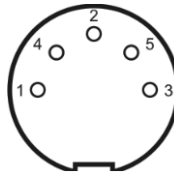
Рисунок 5.4.2.1 – Разъем для внешней синхронизации прибора (со стороны пайки)
