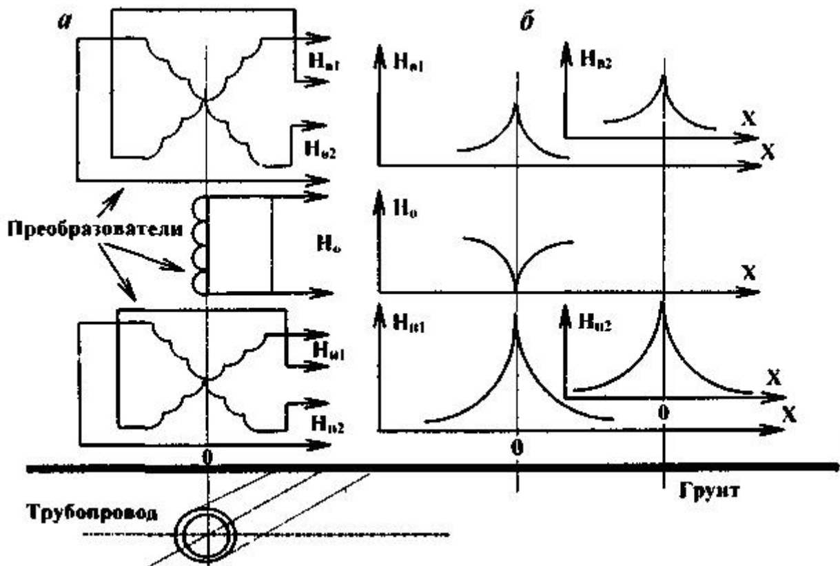
Рисунок 3.1.3.2 - Схематичное расположение преобразователей с отдельными выходными сигналами
