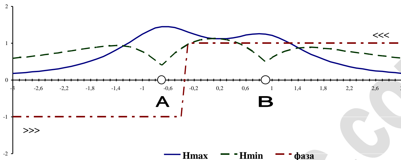
Рисунок 2.12.2.4 – Показания прибора в системе из двух параллельных коммуникаций без интерференции
