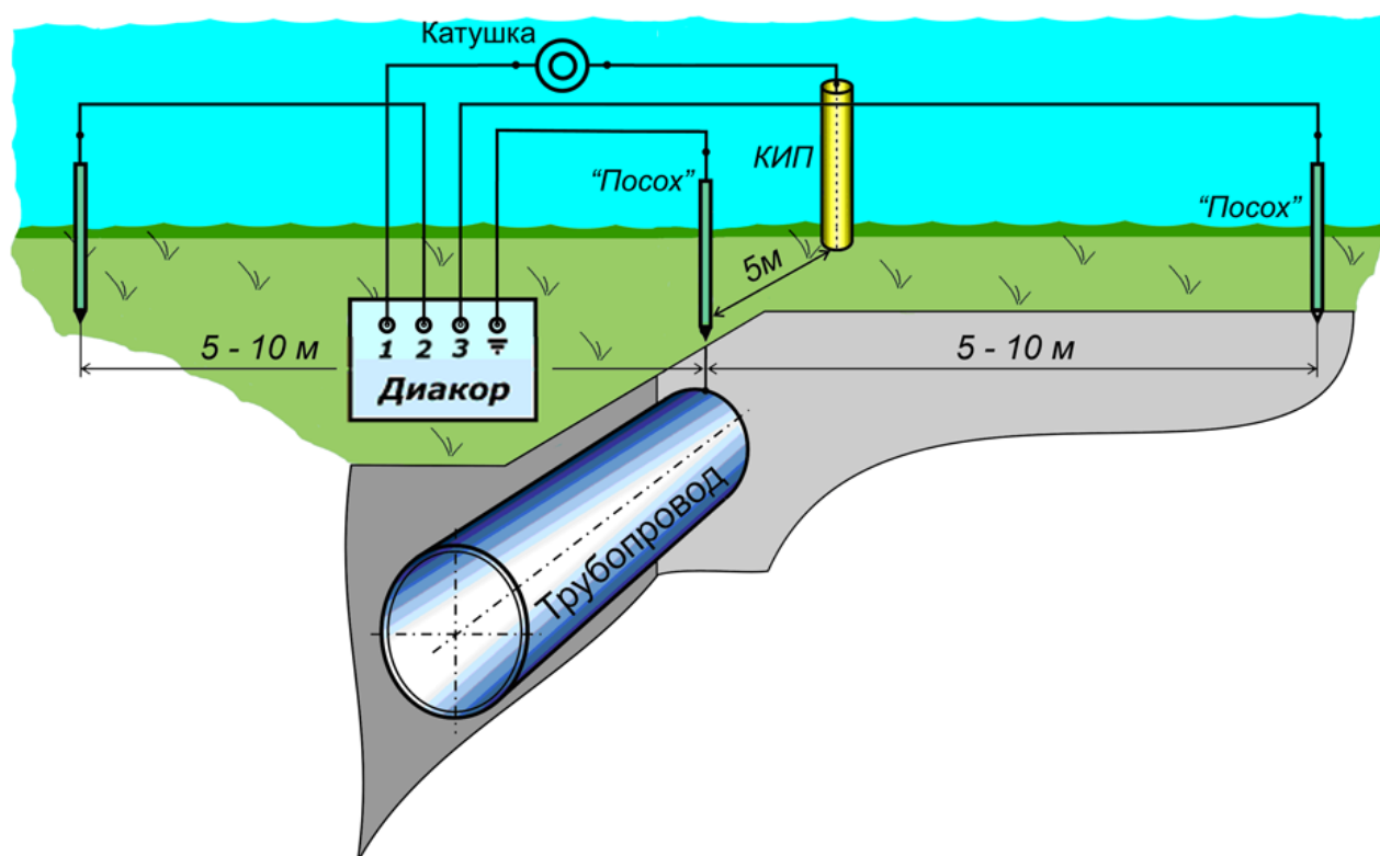
Рисунок 3.1.2.3.2.1 – Трехэлектродный метод
